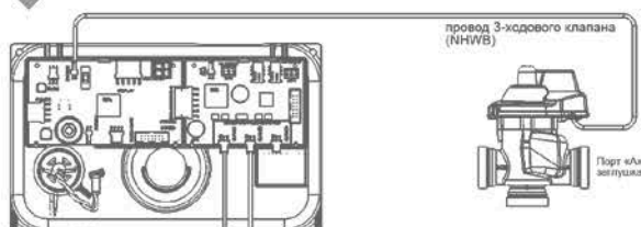
УПР. КЛАПАН 1
