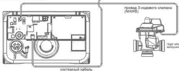
УПР. КЛАПАН 2
